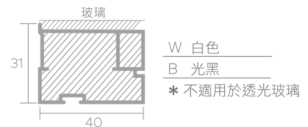
AL506 企柱
