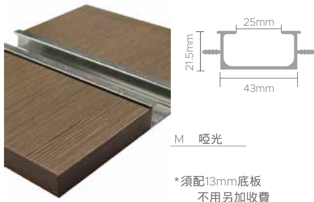
門板封鋁手抽 (1000mm或以下)
