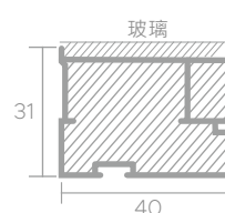
AL506 企柱
